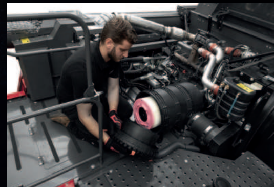
Provera i čišćenje filtera za vazduh
